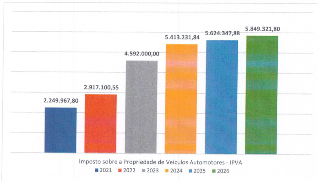
GRÁFICO 3 - EVOLUÇÃO DAS TRANSFERÊNCIAS DA COTA-PARTE IPVA – 2021 A 2026
